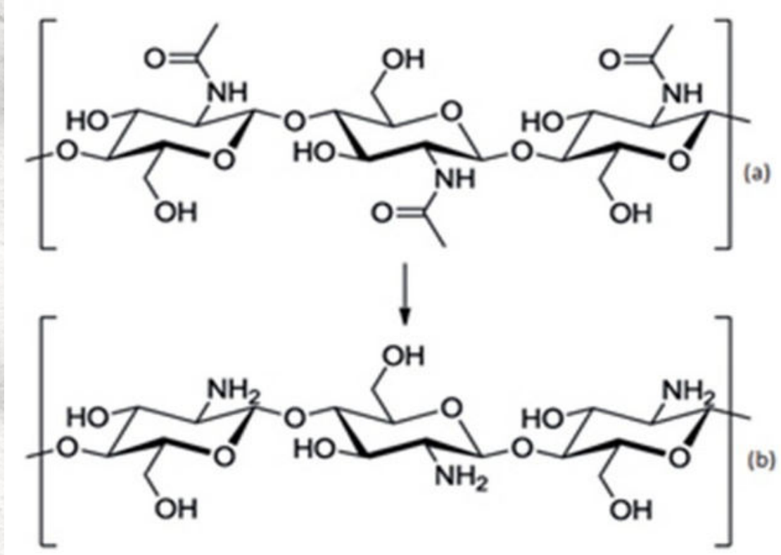
Şekil 1: Kitin (a) ve Kitosan (b) [6]
